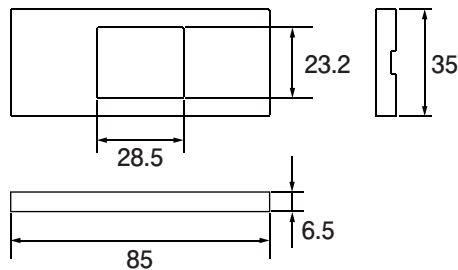
【NCP-9003寸法】
