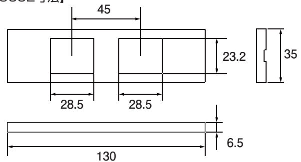
【NCP-9002寸法】
