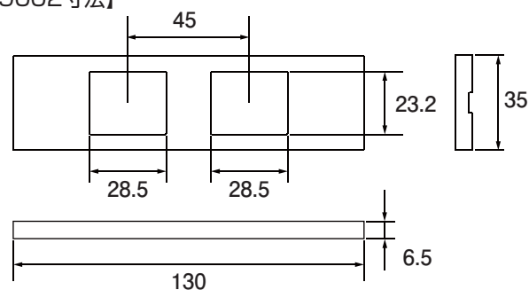
【NCP-9002寸法】
