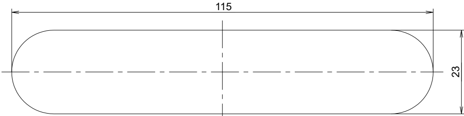
取付穴参考寸法 【取付可能板厚: 6mm以上】
