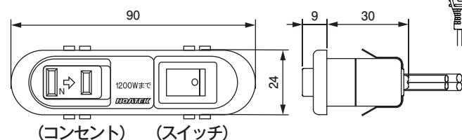
スイッチ連動メスプラグ
