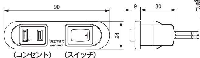
スイッチ連動メスプラグ
